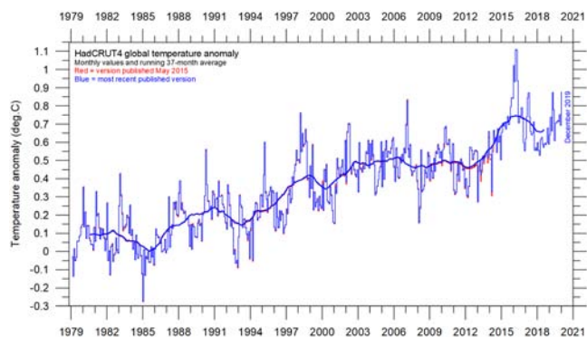
(a) HadCRUT4
