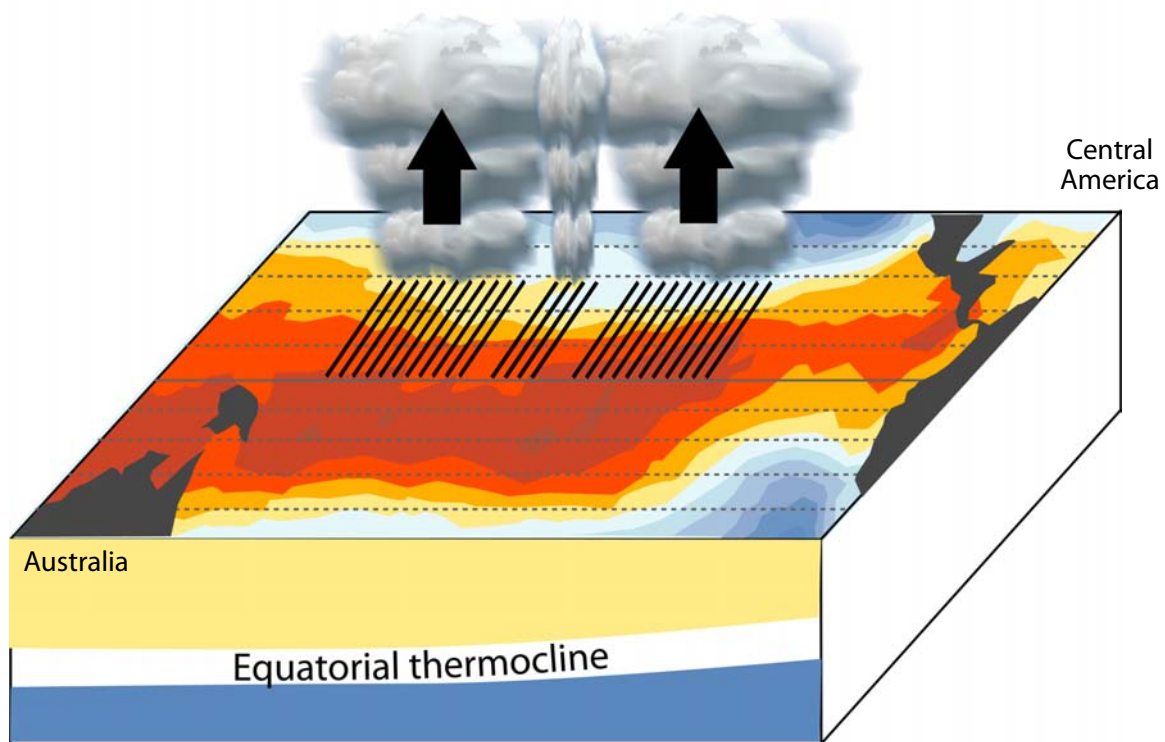
Figure 2: El Niño conditions.
